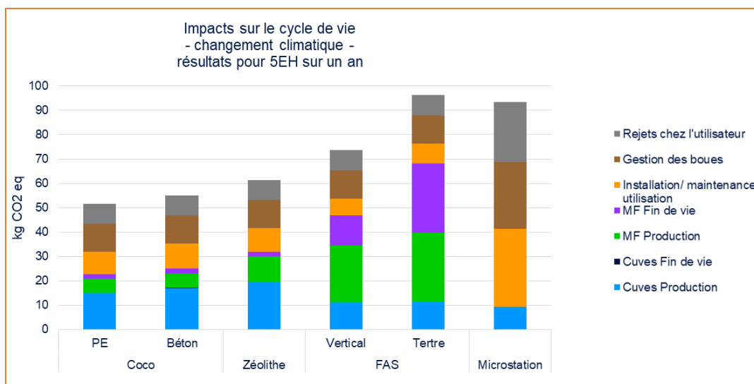
FIGURE 2 – ORIGINE DES IMPACTS ENVIRONNEMENTAUX DU SYSTEME A BASE DE FRAGMENTS DE COCO (CUVE EN PE)
